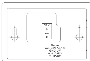
Rys. Nr 10 Widok złączy panelu sterowania
