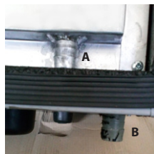
Rys. Nr 5 Syfon na skropliny w RD+ i pochylenie wersji podwieszanej.
