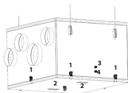
Rys. Nr 4 RD+ w pozycji pracy podwieszanej
