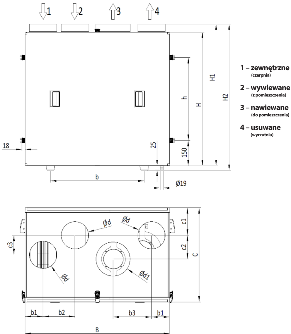
Rys. Nr 1 Kompaktowa centrala RD+
