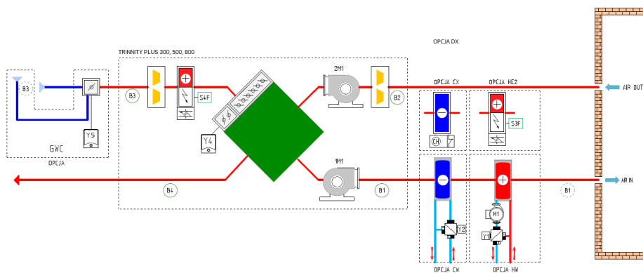
Rys. Nr 2 Schemat automatyki sterownika RD+ uwzględniający sterowanie dodatkowymi urządzeniami.
