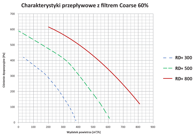
Wykres Nr 1. Ciśnienie dyspozycyjne RD+ 300; RD+ 500; RD+ 800 z filtrem Coarse 60%.
