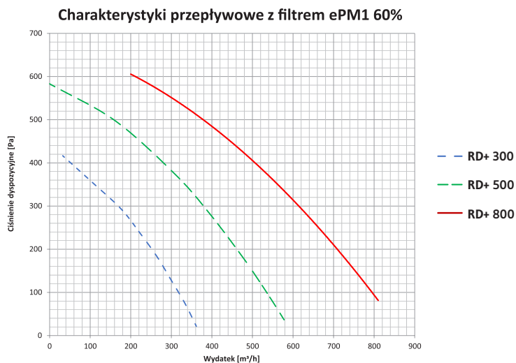
Wykres Nr 2. Ciśnienie dyspozycyjne RD+ 300; RD+ 500; RD+ 800 z filtrem ePM1 60%.
