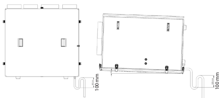
Rys. Nr 5 Syfon na skropliny w RD+ i pochylenie wersji podwieszanej.
