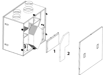
Rys. Nr 7 Sposób wysuwania wymiennika.
